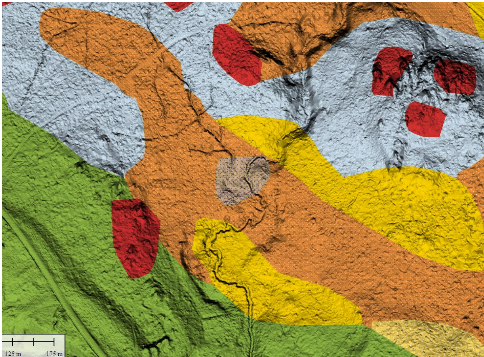
Tinnerbäcken – Exempel på jordartskarta med terrängskuggning
