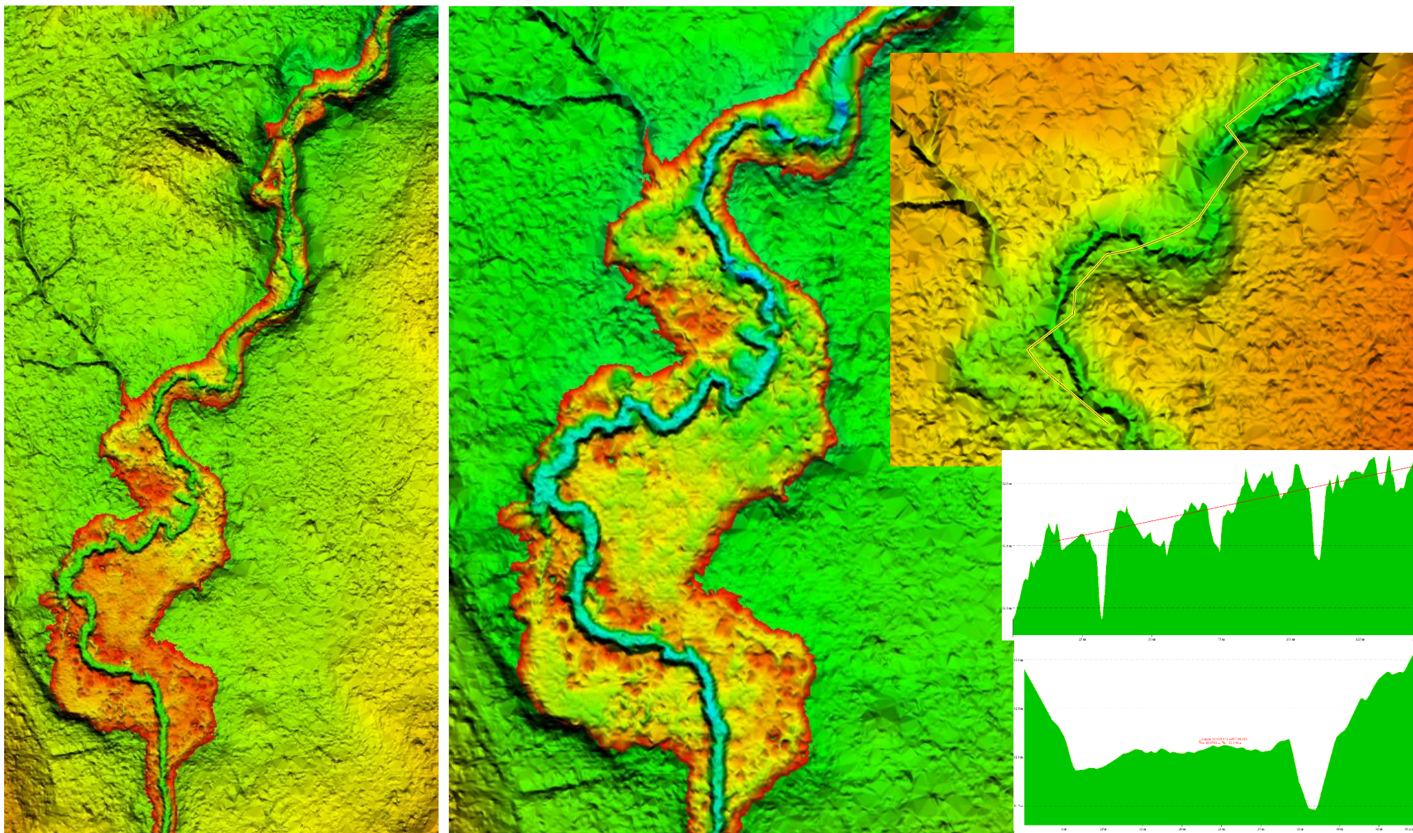
Tinnerbäcken – Exempel på REM, terrängmodell, profil över översvämningsyta samt tvärsektion
